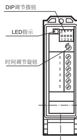
接线端子示意图 RL23-8-H-2000 RLK23-8-H-2000
