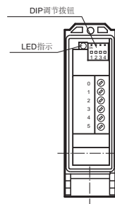
接线端子示意图 RL23-8-H-1000 RLK23-8-H-1000
