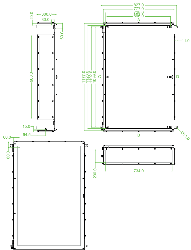
Abbildung/Maßzeichnung zeigt Version mit 4 Flanschplatten.
