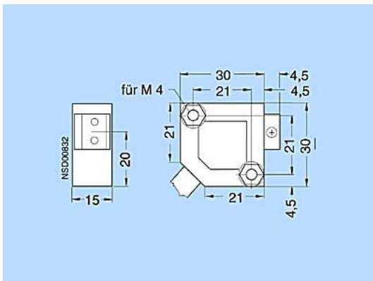
3RG70 13-0...-PF
