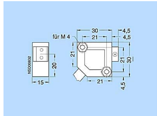
3RG70 13-7...-PF
