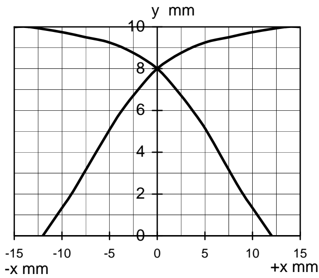
Response characteristics/Ansprechkennlinie:
