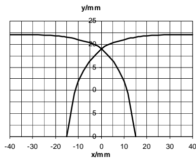
Response characteristics/Ansprechkennlinie:
