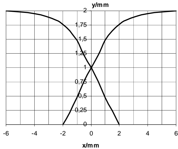
Response characteristics/Ansprechkennlinie:
