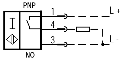
3RG4611-3AG01-PF / 3RG4611-7AG01-PF:
