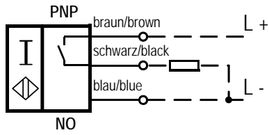
3RG4611-0AG01-PF:
