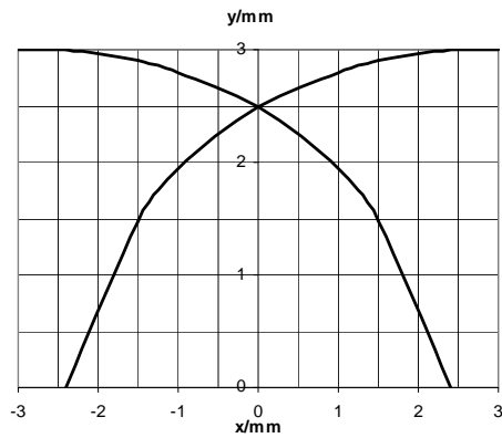
Response characteristics/Ansprechkennlinie:
