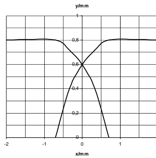
Response characteristics/Ansprechkennlinie:
