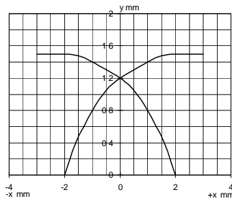
Response characteristics/Ansprechkennlinie:
