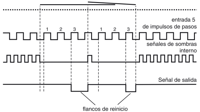
Contar objetos lisos sobre un fondo rugoso: GAB o IAB controlados por impulsos de pasos externos (en el ejemplo está ajustado a n = 3). Se cuentan los flancos de reinicio.
