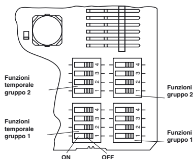
Posizione degli interruttori DIP
