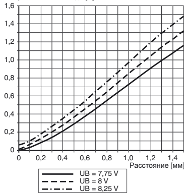
Характеристика срабатывания Напряжение на выходе [В]
