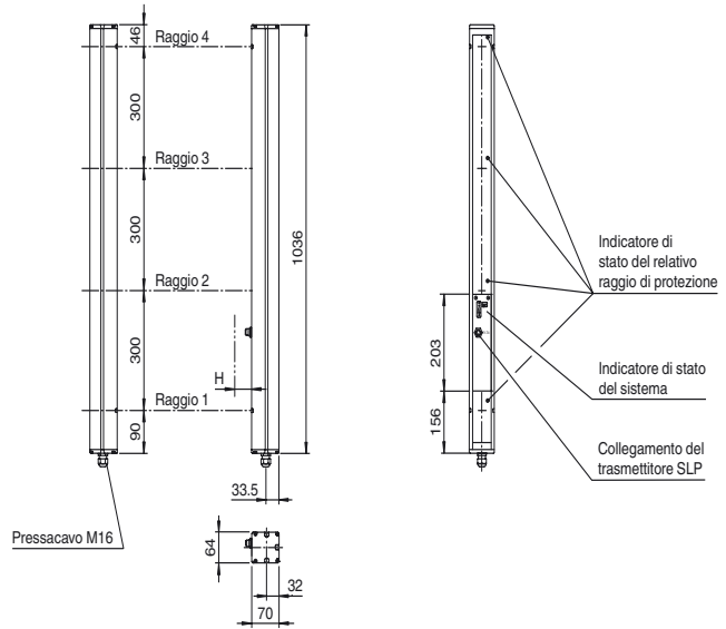
Unità di trasmissione SLP...-4-T Ricevitore SLPC...-4-R
