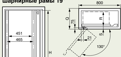
Шарнирные рамы 19"
