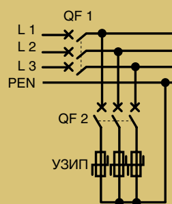
Трехфазная система
