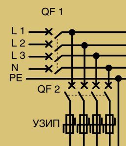
Трехфазная система
