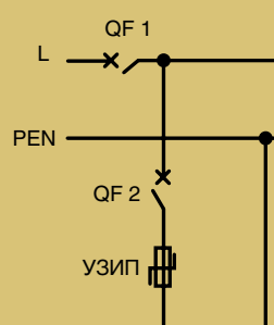
Однофазная система
