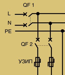
Однофазная система
