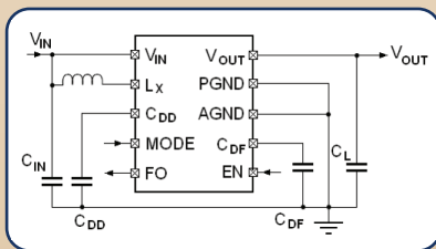
IXD2135 schematic
