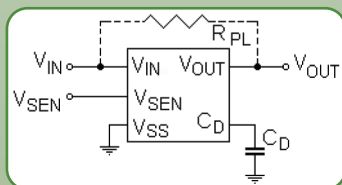
IXD5118 schematic
