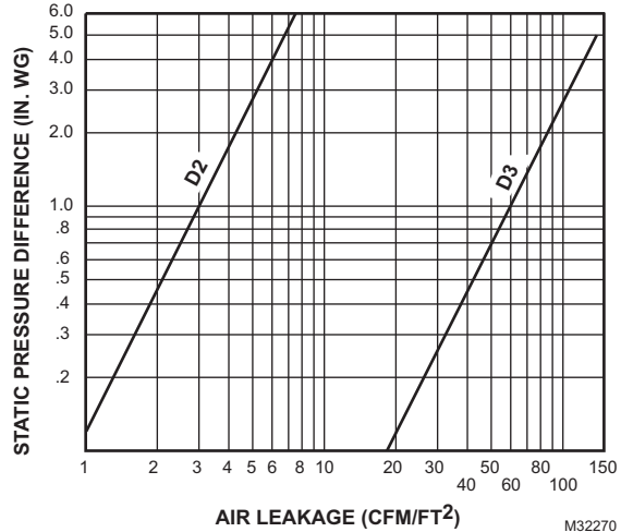
Fig. 6. D2, D3 leakage data.
