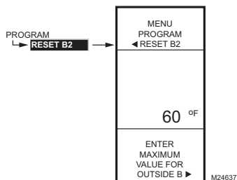
Fig. 69. Programmation - Point de consigne maximal du capteur B.
