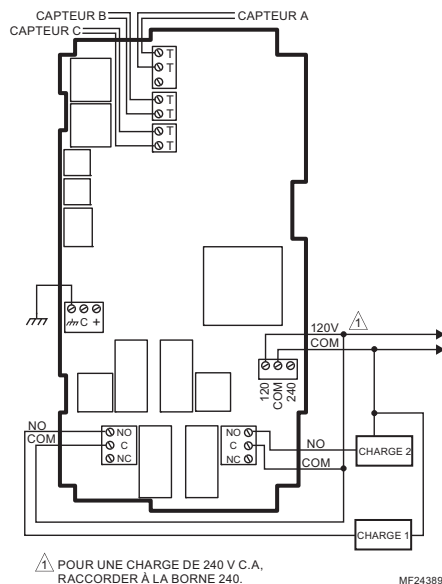
Fig. 10. Raccordement électrique d'un régulateur à deux étages - 120 ou 240 V c.a. (entrée de 120 V c.a. et charge de 120 V c.a.).
