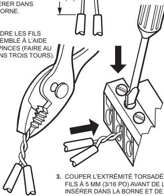
Fig. 6. Raccordement de deux fils ou plus au bornier.
