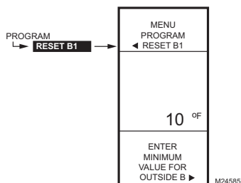
Fig. 67. Programmation - Point de consigne minimal du capteur B.
