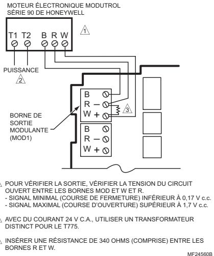
Fig. 18. Raccordement d'un moteur Modutrol série 90.
