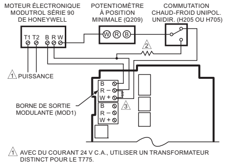
Fig. 18. Raccordement d'un moteur Modutrol série 90.
