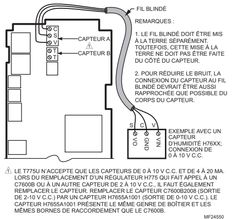
Fig. 5. Raccordement du capteur – Connexion d'un fil blindé à trois brins de la borne du capteur A au capteur de 0 à 10 V c.c. (illustré : capteur d'humidité H76XX).
