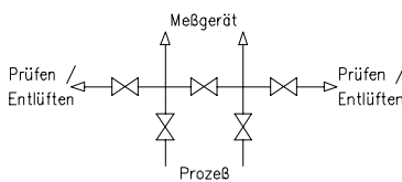
Schaltschema 1
