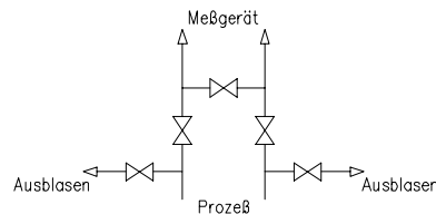
Schaltschema 2
